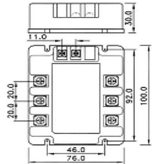
Габаритно-установочные размеры (мм)
